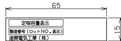
定格銘板詳細
